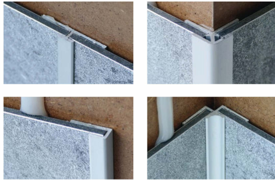
Zubehör: z.B. Profile in vier verschiedenen Farben
