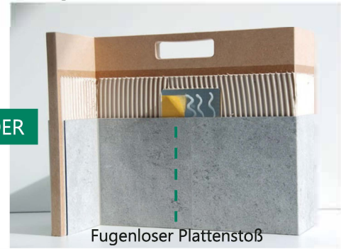
Montage II: 2K-Kleber
